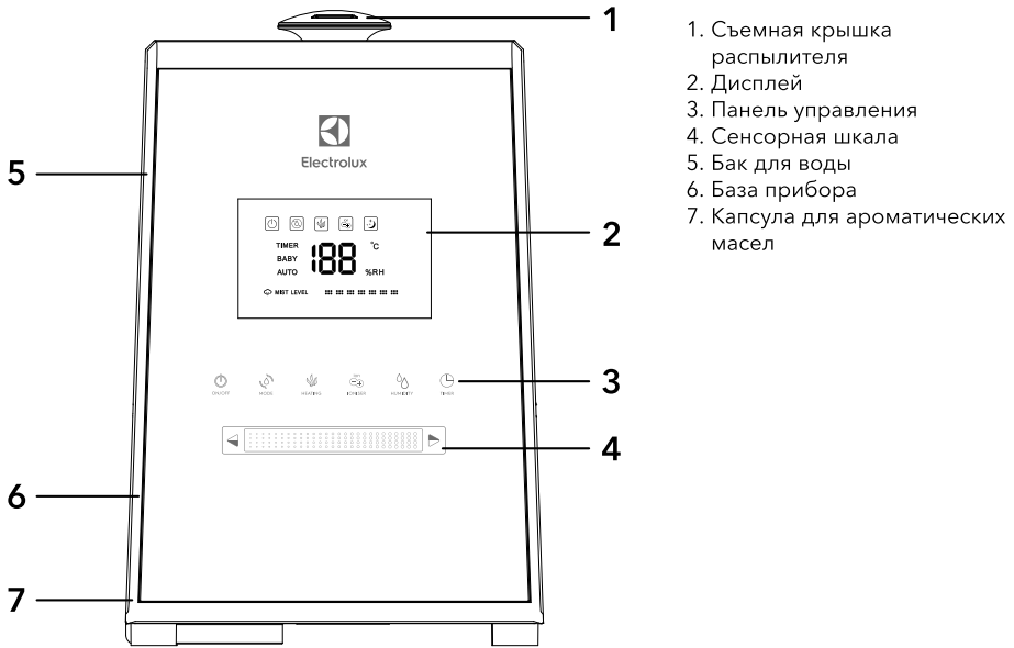
Рис. 1 Описание прибора
