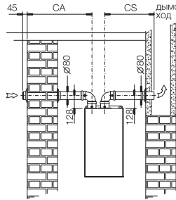
Воздухозабор через стену, дымоотвод в дымоход
