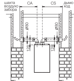
Воздухозабор из вентиляционной шахты, дымоотвод в дымоход
