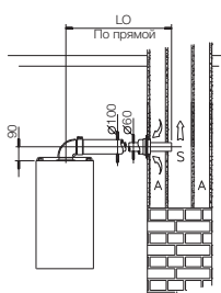
Горизонтальный коаксиальный дымоход
