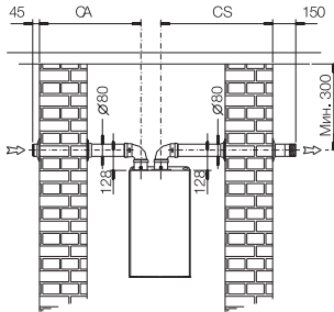
Воздухозабор и дымоотвод через стену
