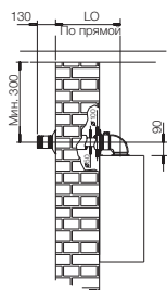
Горизонтальный коаксиальный дымоход
